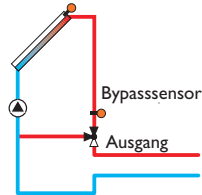
Typ Ventil
